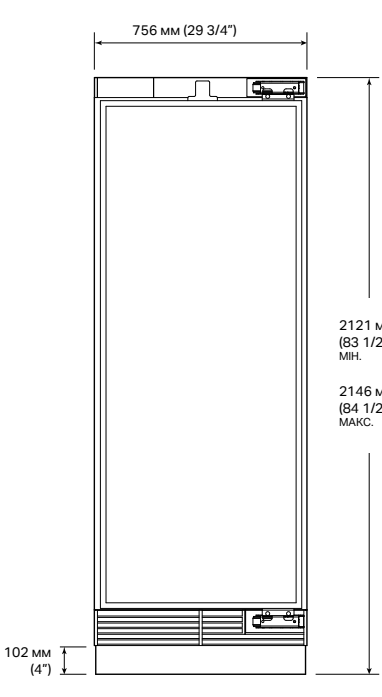
ВИД СПЕРЕДУ
