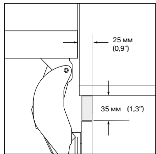
ВІДКРИТТЯ ДВЕРЦЯТ НА 90°
