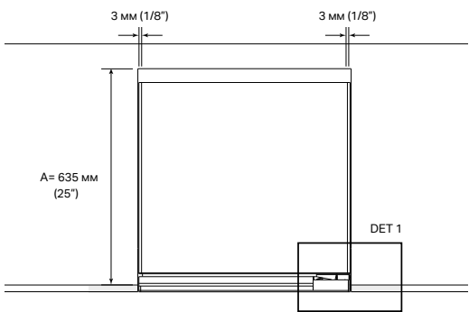
DET 1
