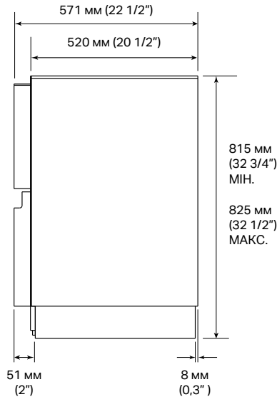
ВИД ЗБОКУ
