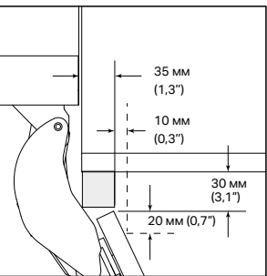
ВІДКРИТТЯ ДВЕРЦЯТ НА 115°
