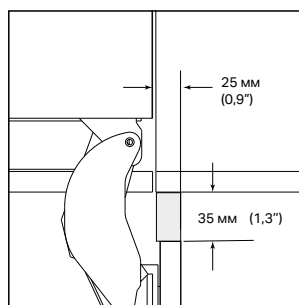
ВІДКРИТТЯ ДВЕРЦЯТ НА 90°
