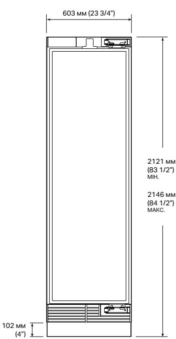
ВИД СПЕРЕДУ
