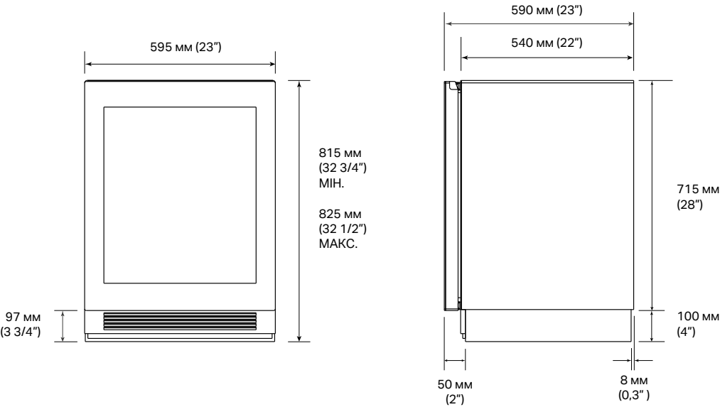
ВИД СПЕРЕДУ
