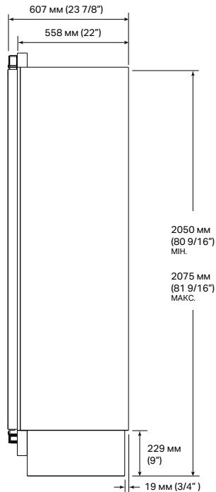
ВИД ЗБОКУ
