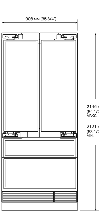
ВИД СПЕРЕДУ
