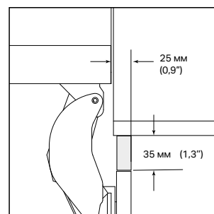
ВІДКРИТТЯ ДВЕРЦЯТ НА 115°
