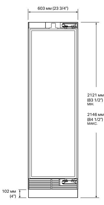
ВИД СПЕРЕДУ
