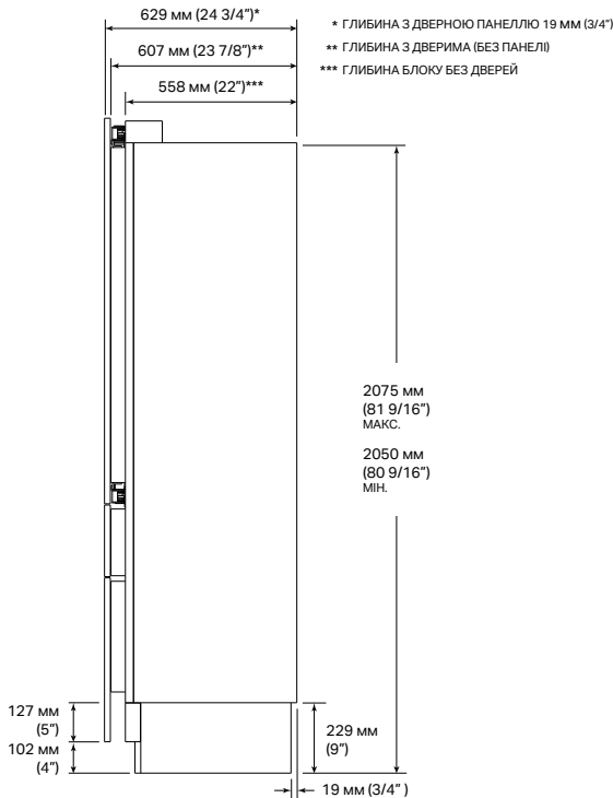
ВИД ЗБОКУ
