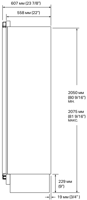
ВИД ЗБОКУ
