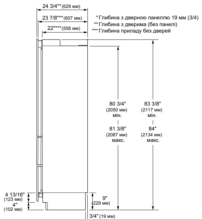
ВИД ЗБОКУ
