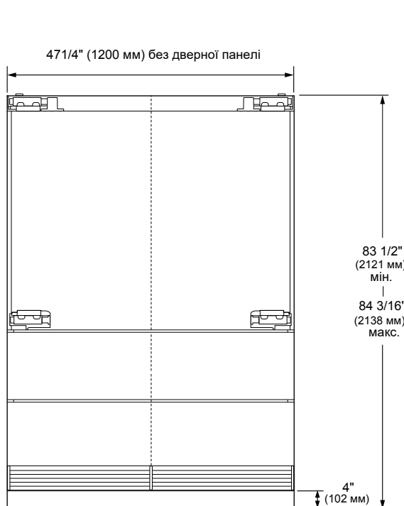
ВИД СПЕРЕДУ
